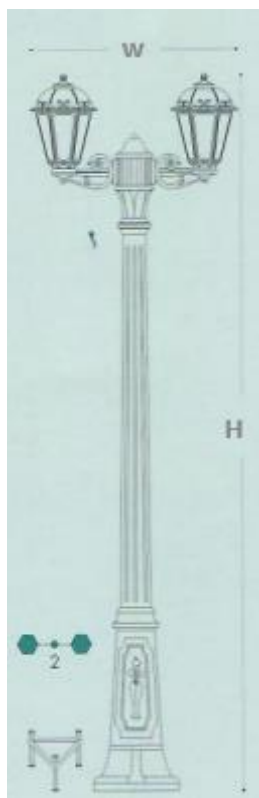
Εικόνα 1. Φωτιστικός ιστός παραδοσιακού τύπου
